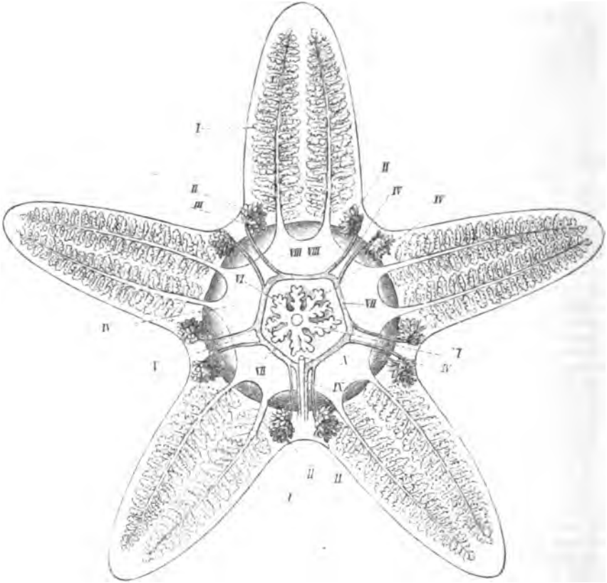
C. 1852. Soustava zaživací a pohlavní ústrojí hvězdice (schematicky).
